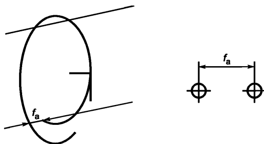
Рисунок 1 — Спиральная укладка проволоки
